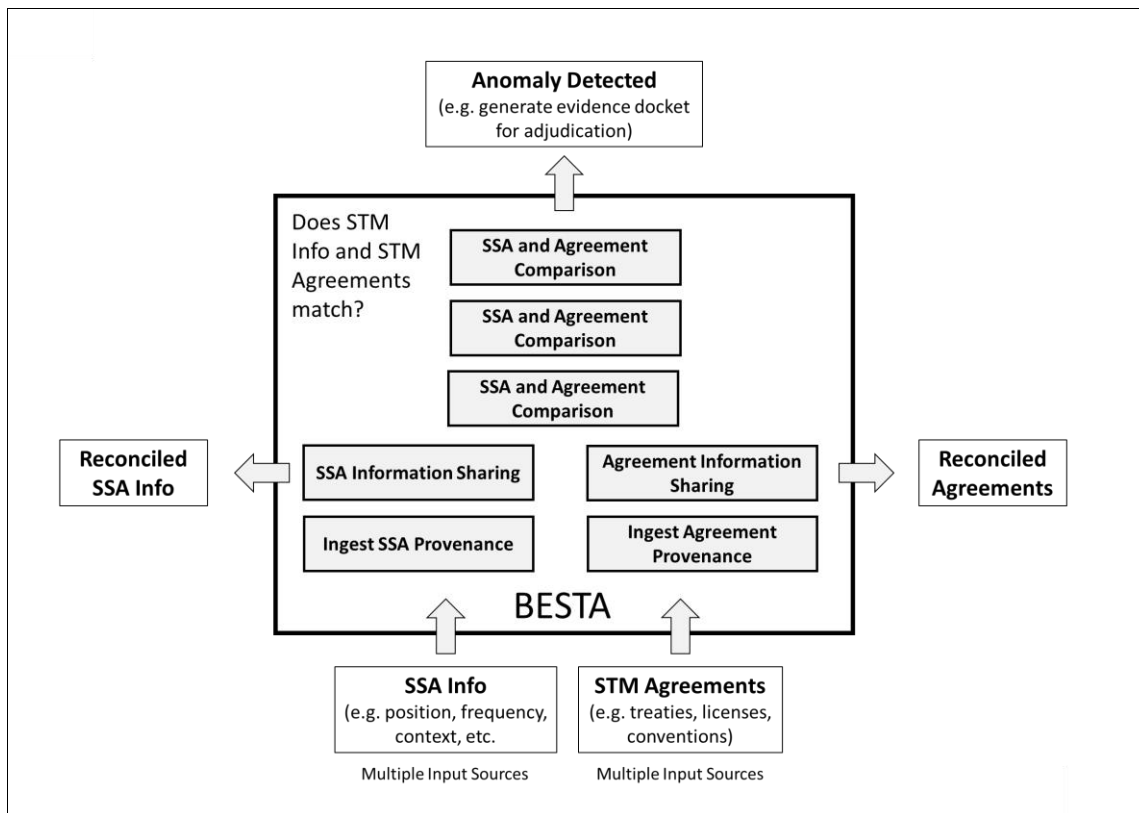
Fig. 7 BESTA Internals
